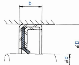
VAJ type
