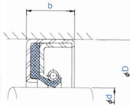
SA1J type
